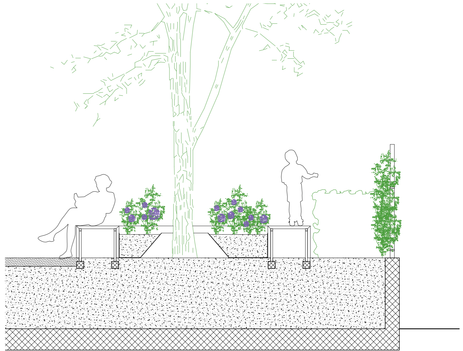
Coupe ponton
