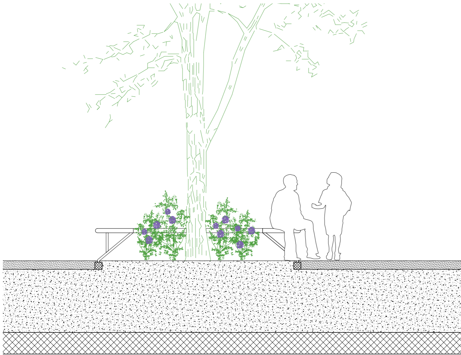
Coupe banc
